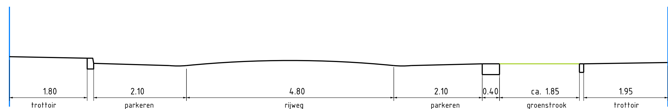
Principe profiel (van Flintdijk 172 tot Flintdijk 200)
