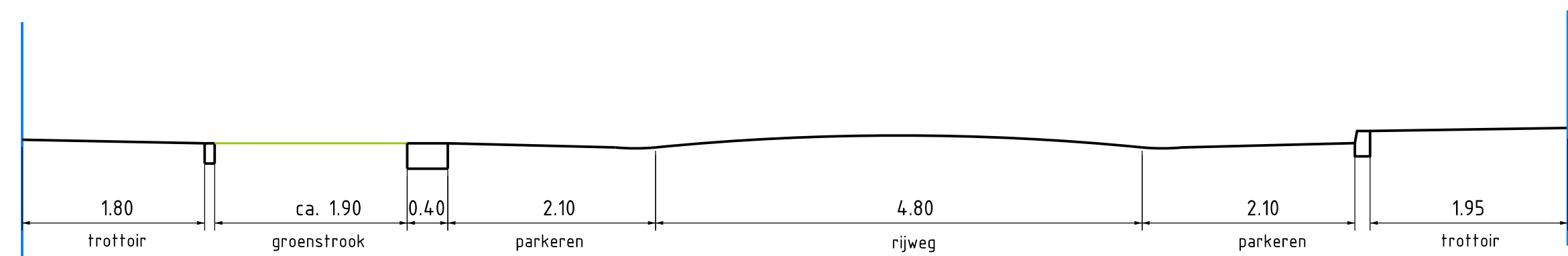
Principe profiel (van Flintdijk 202 tot Flintdijk 218)
