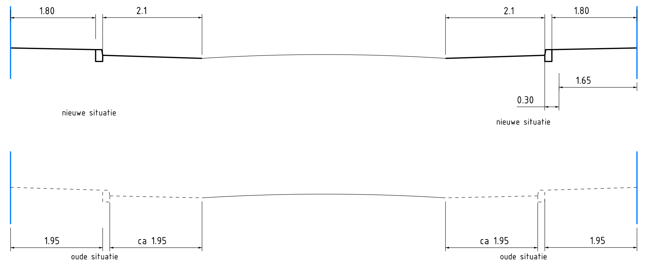
Principe profiel (van Flintdijk 2 tot Flintdijk 170)
