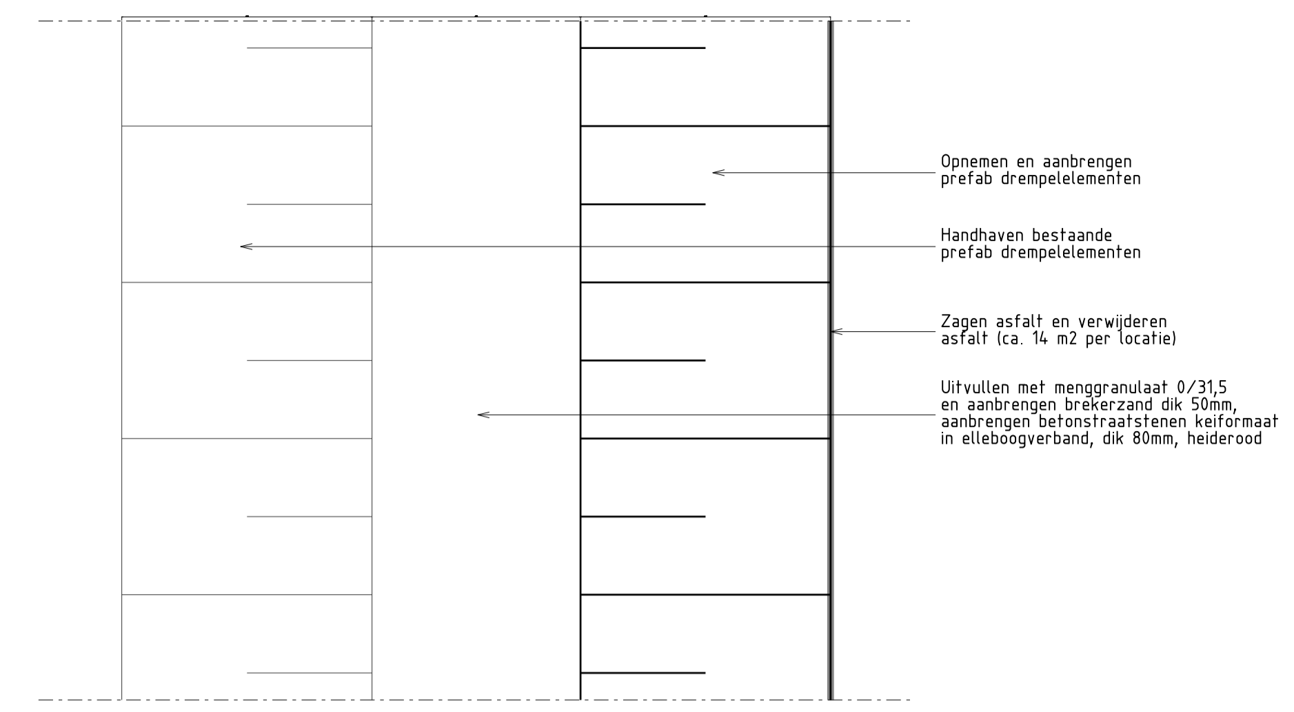
Principedetail drempe Elisadonk Schaal 1:50
