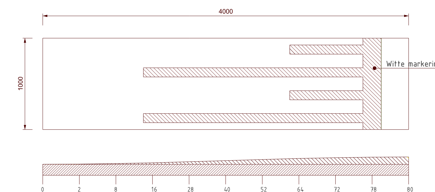
Verkeersdrempel 60KM/H in asfalt
